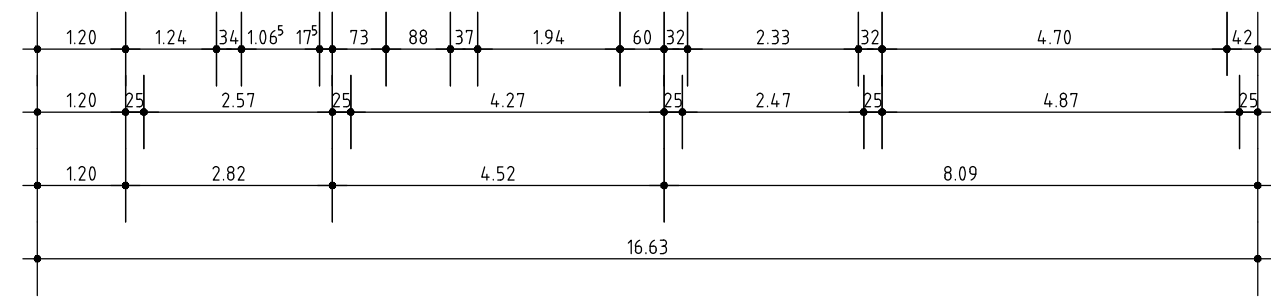
GRUNDRISS NEBENGEBÄUDE
